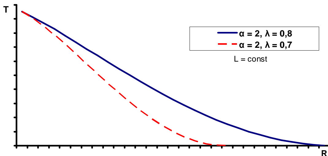
Рис. 4. График PPF при IRS в секторе T и DRS в секторе R
